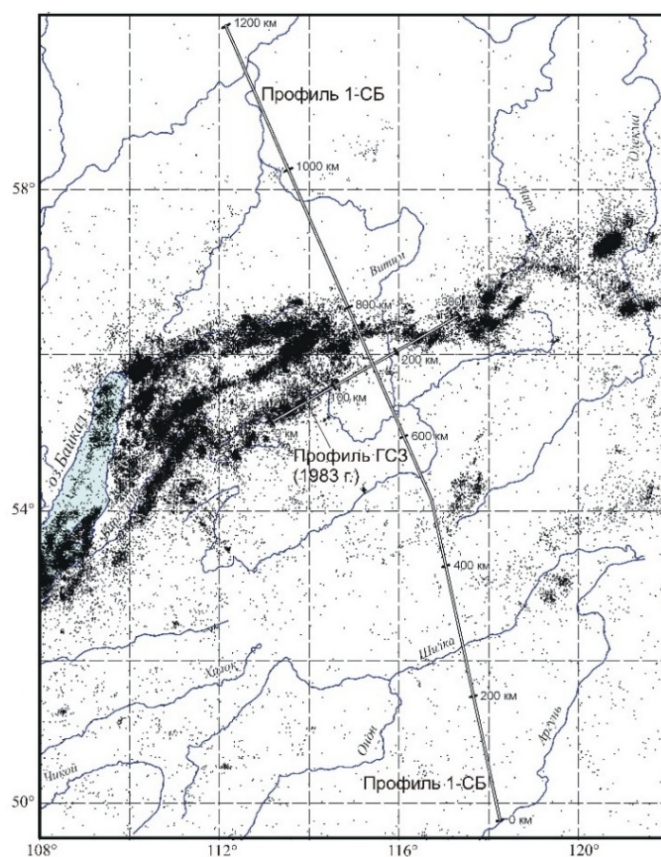
Рис. 1. Схема тектонического районирования согласно [12] (а) и карта эпицентров землетрясений с Kp \geq 6.6 за 40 лет с 1975-2014 гг. (б) в полосе опорного профиля 1-СБ (Восточный участок)
