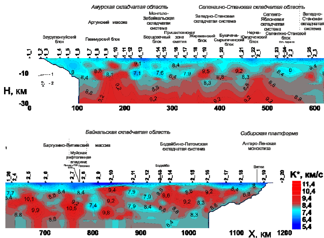
Рис. 3. Распределение параметра K^* = V_p/(\gamma - 1) (где \gamma = V_p/V_s ) в земной коре и верхней мантии на профиле 1-СБ (Восточный участок): 1 – изолинии параметра K^* , в км/с; 2 – источники возбуждения (1-Забайкальский фрагмент, 2-Байкало-Патомский фрагмент).
