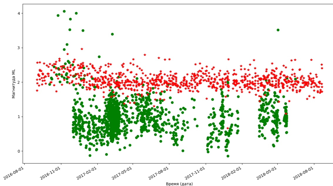
Рис. 3. Временная развертка сейсмического процесса в зоне активизации.
