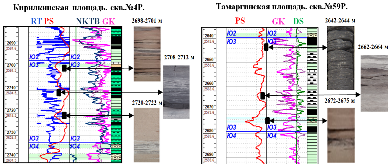
Рис. 5. Литофациальная характеристика континентальных разрезов IV типа
