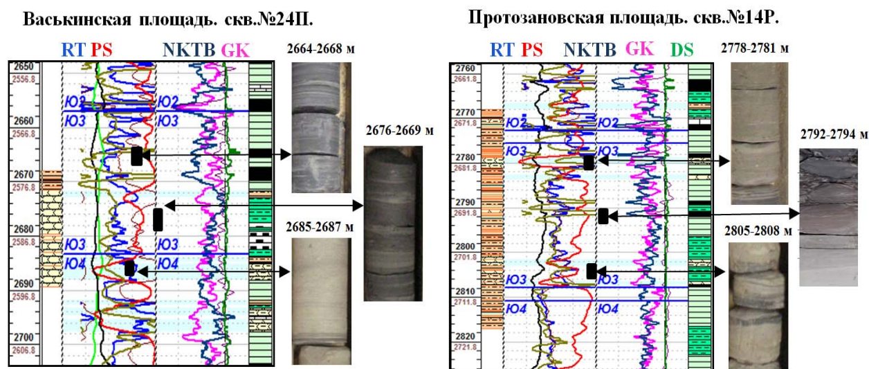
Рис. 4. Литофациальная характеристика континентальных разрезов III типа
