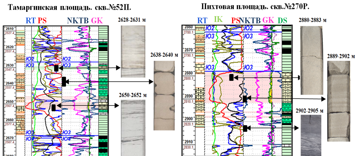
Рис. 3. Литофациальная характеристика континентальных разрезов II типа
