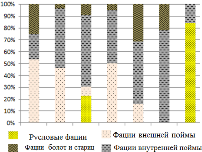
Пример распределения фаций по керну в скважинах Уватского проекта
