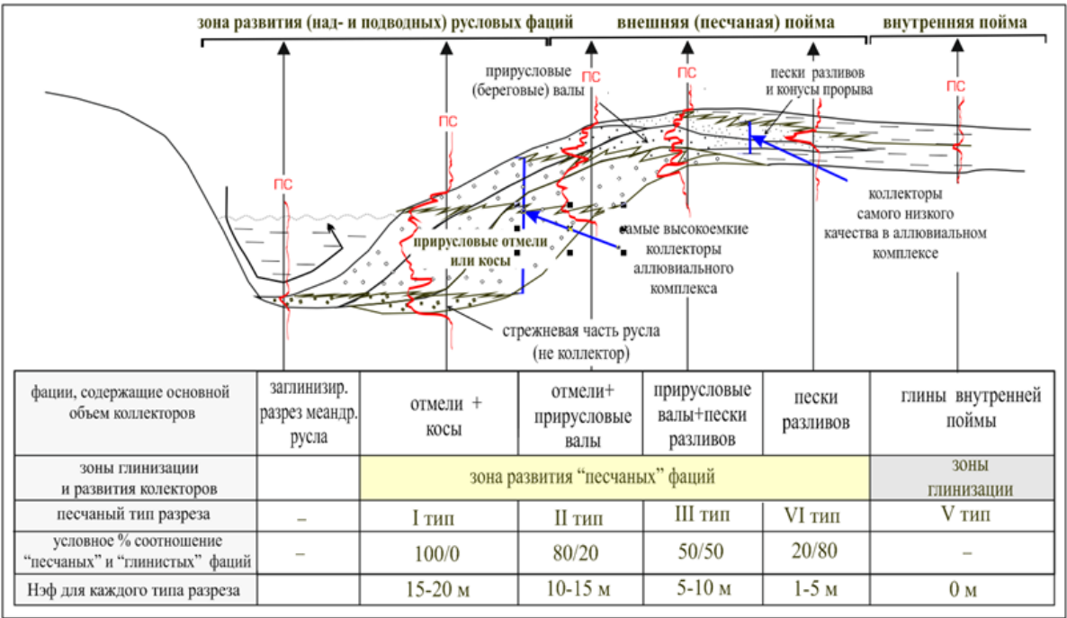
Пример распределения фаций по керну в скважинах Уватского проекта
