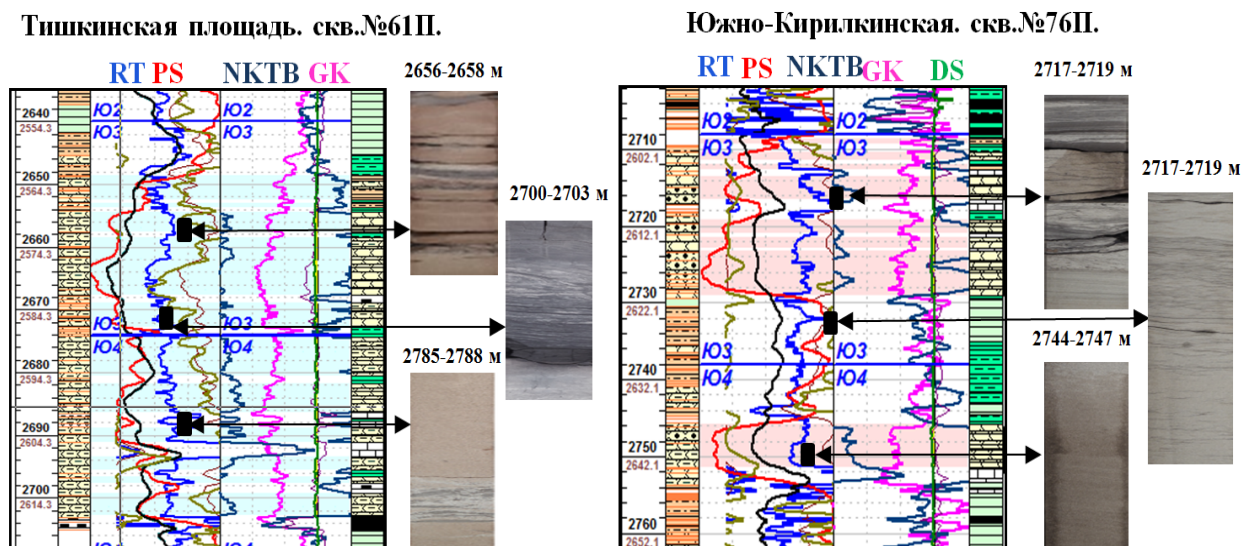
Рис. 2. Литофациальная характеристика континентальных разрезов I типа
